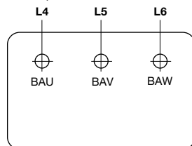
Figure 3Q - Schémas de raccordement moteur et frein
