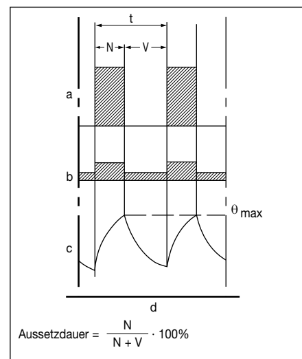
Abbildung 3G - Betrieb S6
