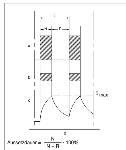
Abbildung 3D - Betrieb S3
