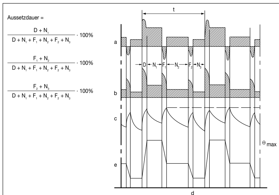
Abbildung 3I - Betrieb S8
