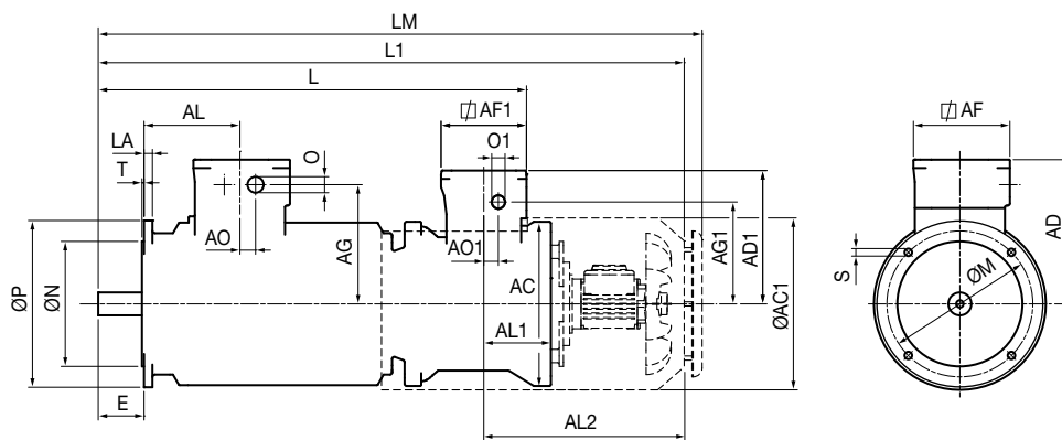
IM B5
