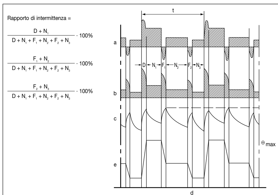
Figura 3I - Servizio S8
