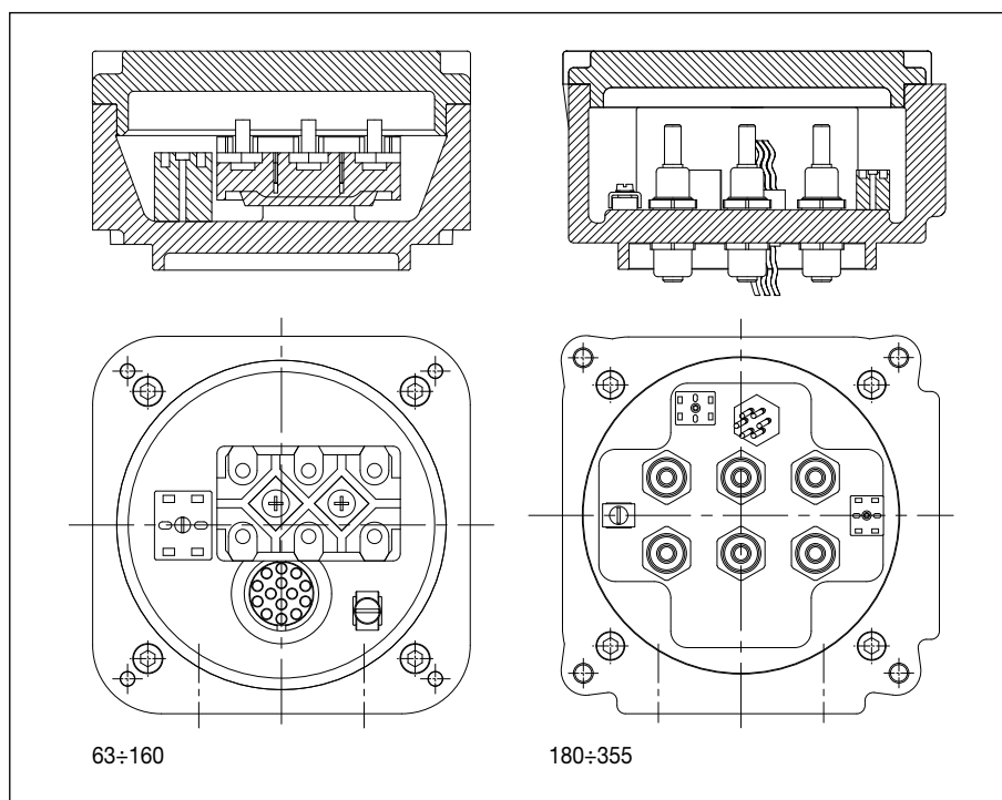
Figure 20 - Boîte à bornes moteurs standard version Ex d, groupe IIB/IIC
