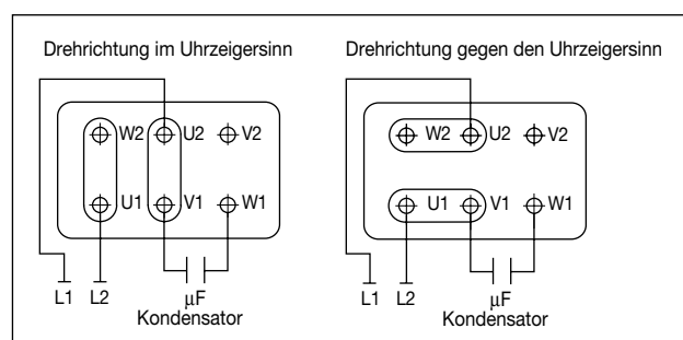
Abbildung 3P - Schaltungsschema für Einphasenmotoren
