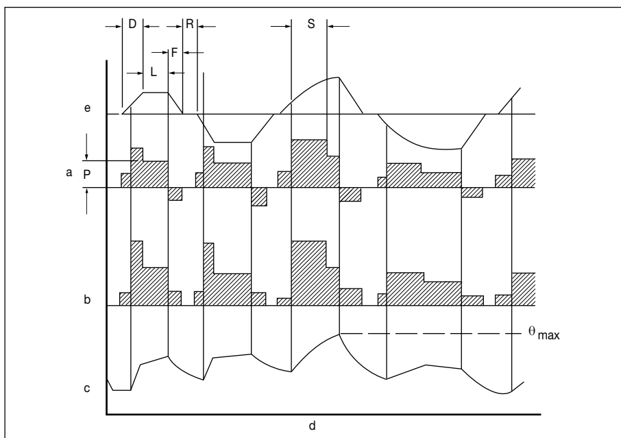
Abbildung 3L - Betrieb S9
