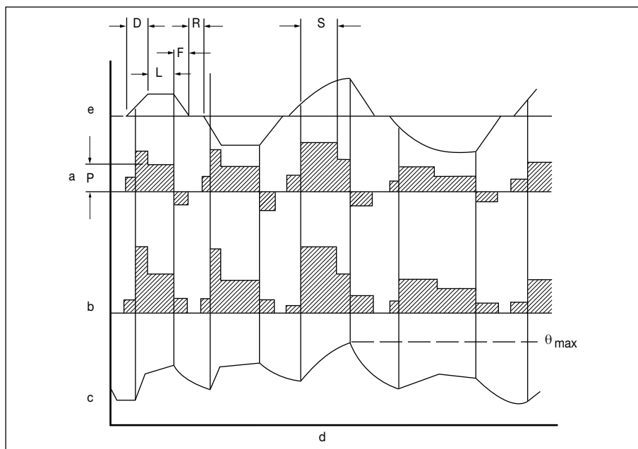
Figura 3L - Régimen S9
