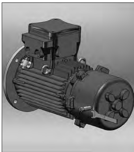
Figura 2E - Sblocco manuale (opzionale su richiesta) per motori 71÷160 non ventilati
