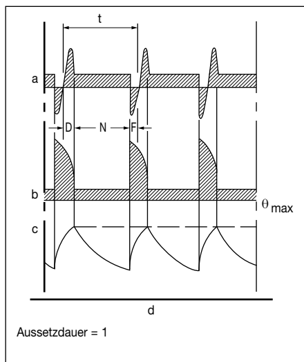
Abbildung 3H - Betrieb S7
