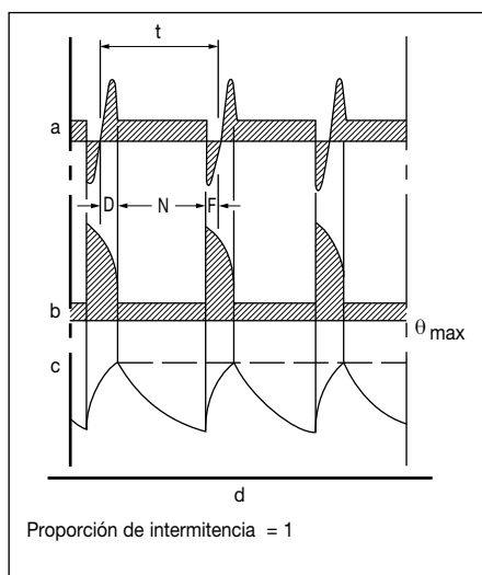
Figura 3H - Régimen S7
