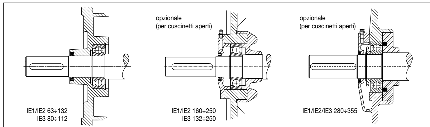
Figura 2H - Cuscinetti a sfera - DE (anteriore)
