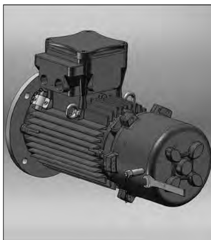
Figure 2E - Déblocage manuel (option sur demande) pour des moteurs 71÷160 non ventilé
