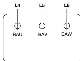
Figura 3Q - Schemi di collegamento motore e freno
