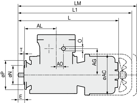
IM B14
