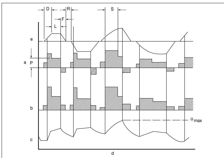
Figura 3L - Servizio S9
