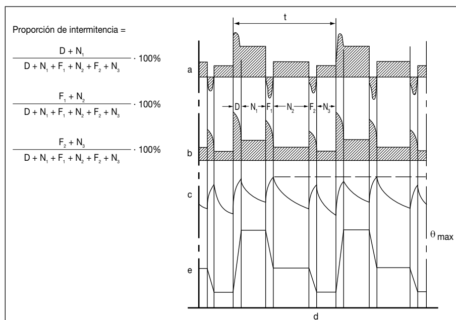
Figura 3I - Régimen S8
