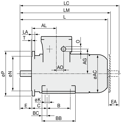
IM B35
